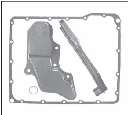
RE4R03A Infiniti/Nissan 300ZX w Turbo 90-97 Q45 90-98
