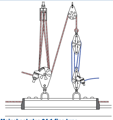
6:1 Mainsheet plus 24:1 fine tune
